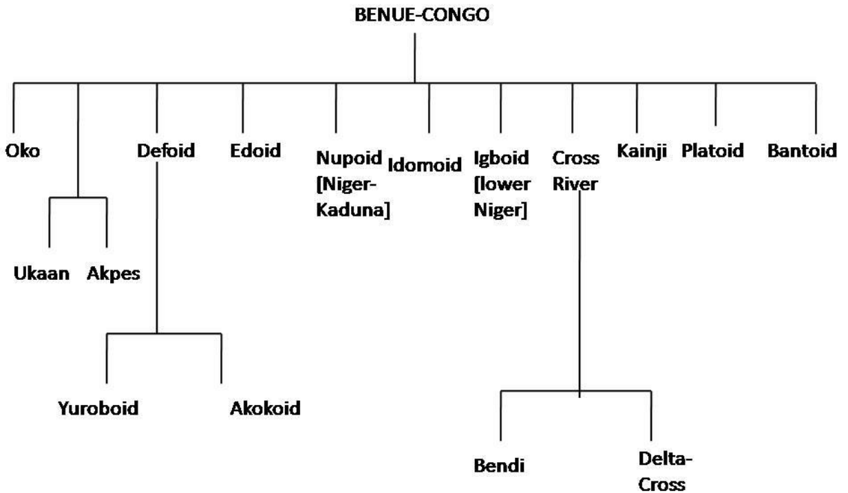
Àwòrán 2: Àwòrán igi tó n sàfihàn mọ̀lẹ̀bí èdè Benue-Congo
